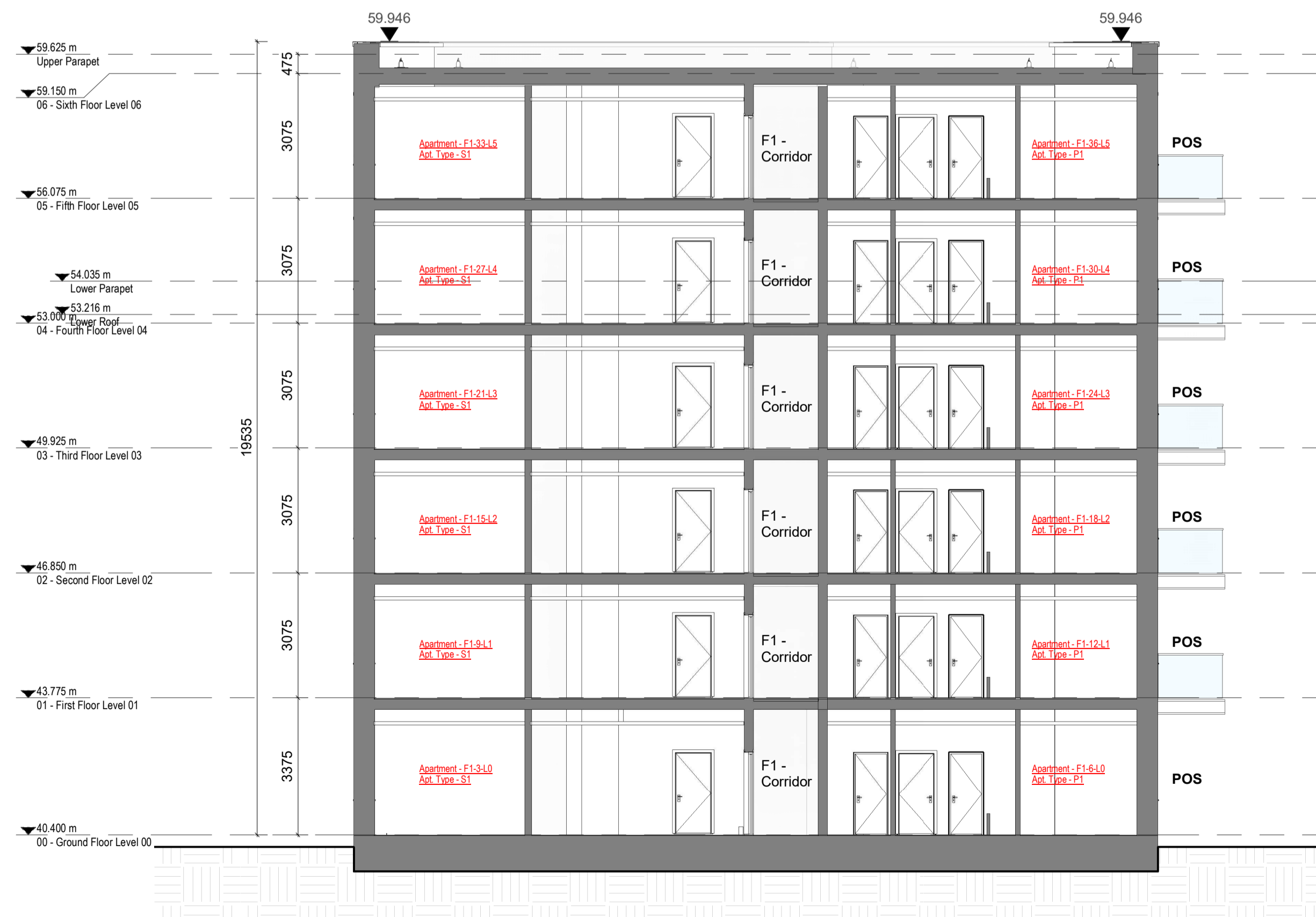
2 GA - Section CC 1 : 100
